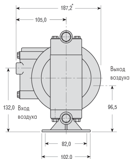
Вид сбоку
