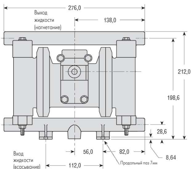
Вид спереди
