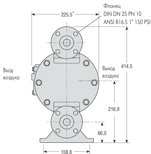
Вид сбоку
