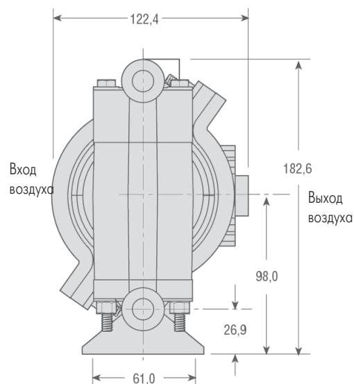
Вид сбоку
