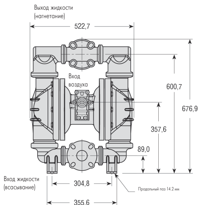
Вид спереди
