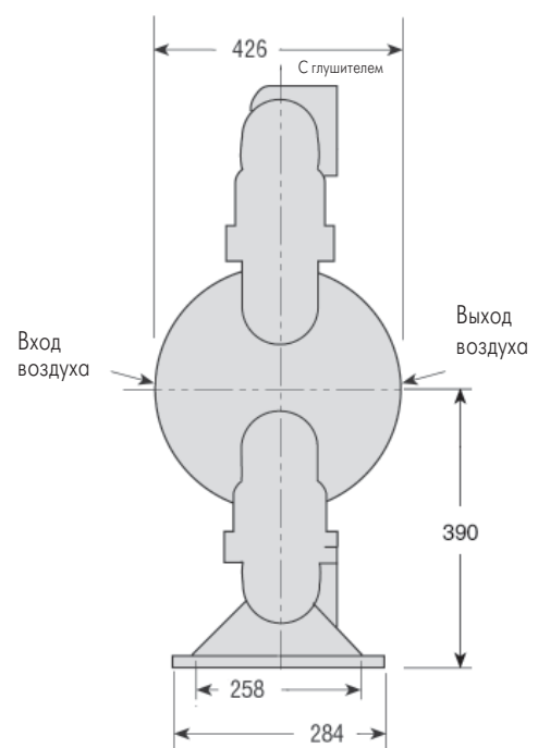
Вид сбоку
